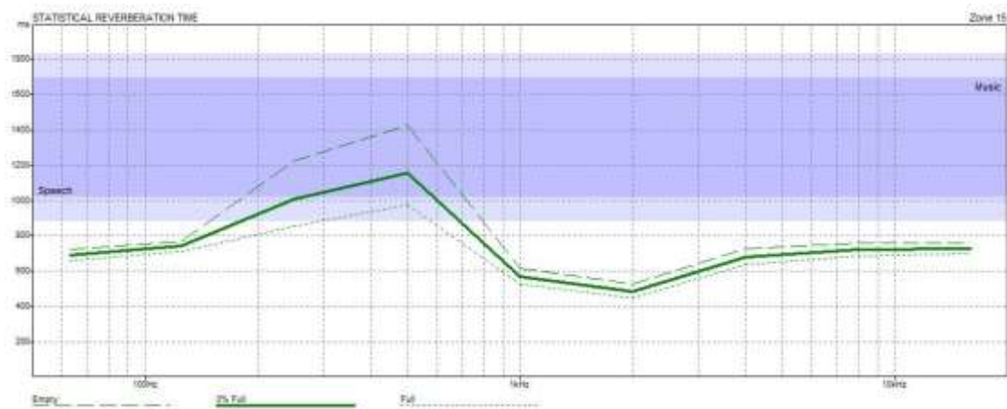
Gambar 7 Grafik waktu dengung dengan occupancy sebesar 0%,50% dan 100% setelah pergantian material
